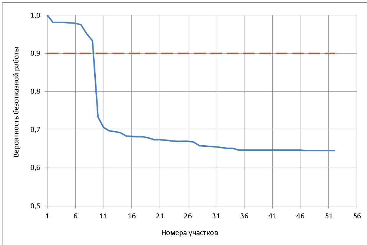
Рисунок 3.4 – ВБР относительно ТК потребителя «ПТ-пл.Революция, 7 восток» тепловых пунктов зоны Сормовской ТЭЦ (расчетный путь 1-2)
